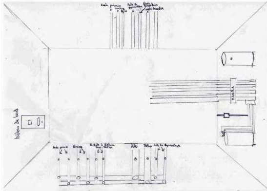
Stockmar : le schéma de chauffage
