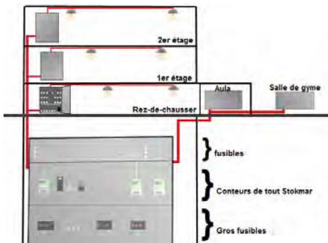
Stockmar : le schéma électrique
